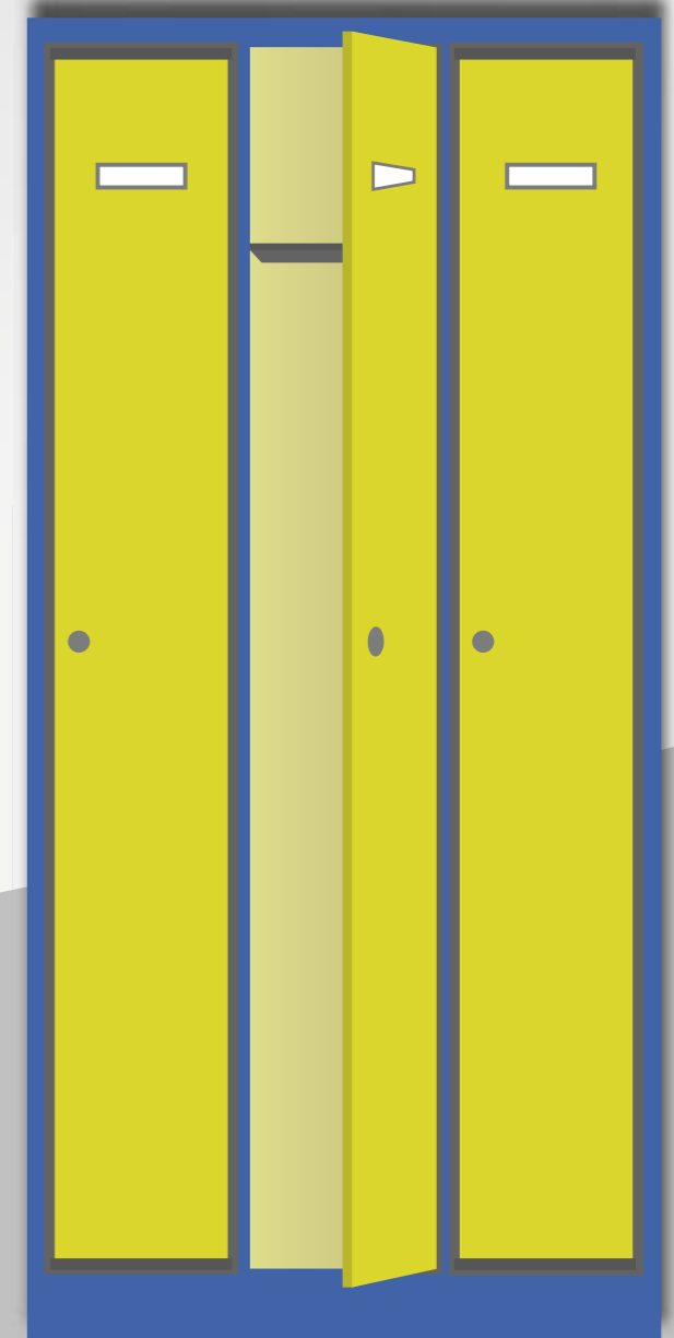
Zeichnung: Rigi Standard, Breite 900 x Tiefe 500 x Höhe 1750 mm
